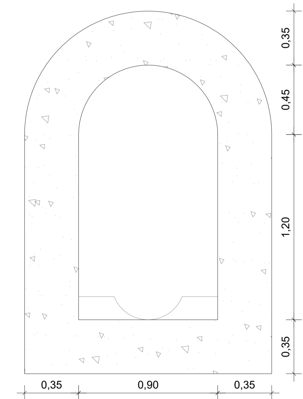
SECCIÓ A-A ESCALA A3 1:30 ESCALA A1 1:15
