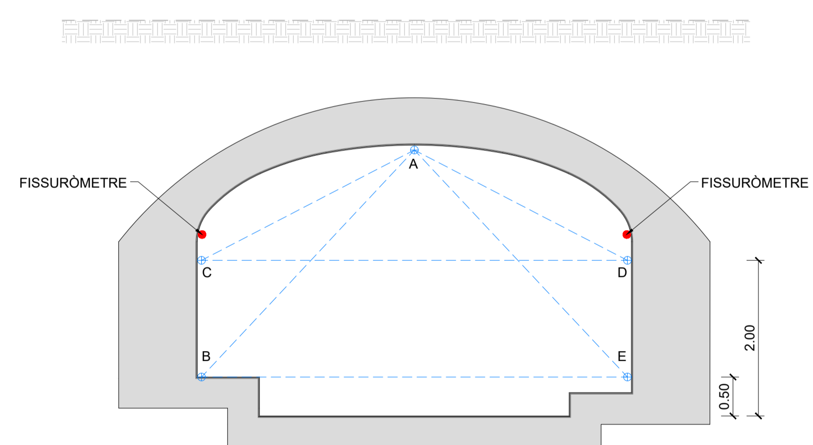
SECCIÓ A-A
