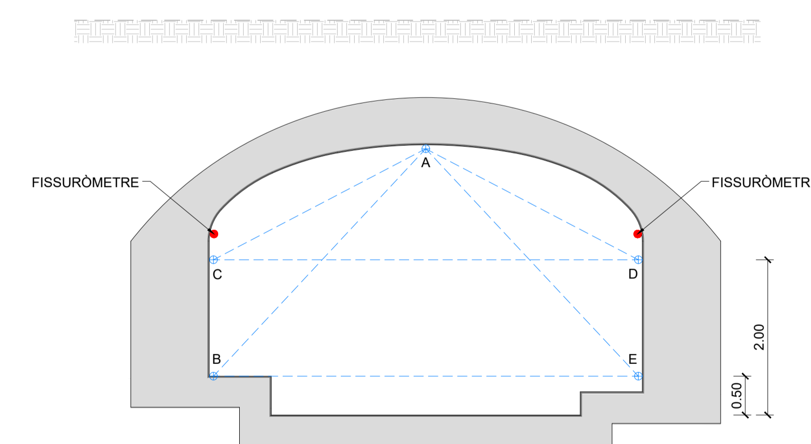
SECCIÓ C-C
