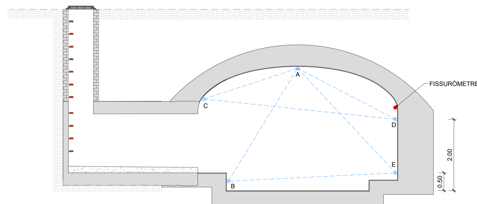
SECCIÓ B-B
