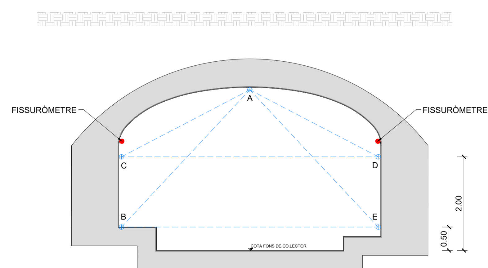
SECCIÓ A-A
