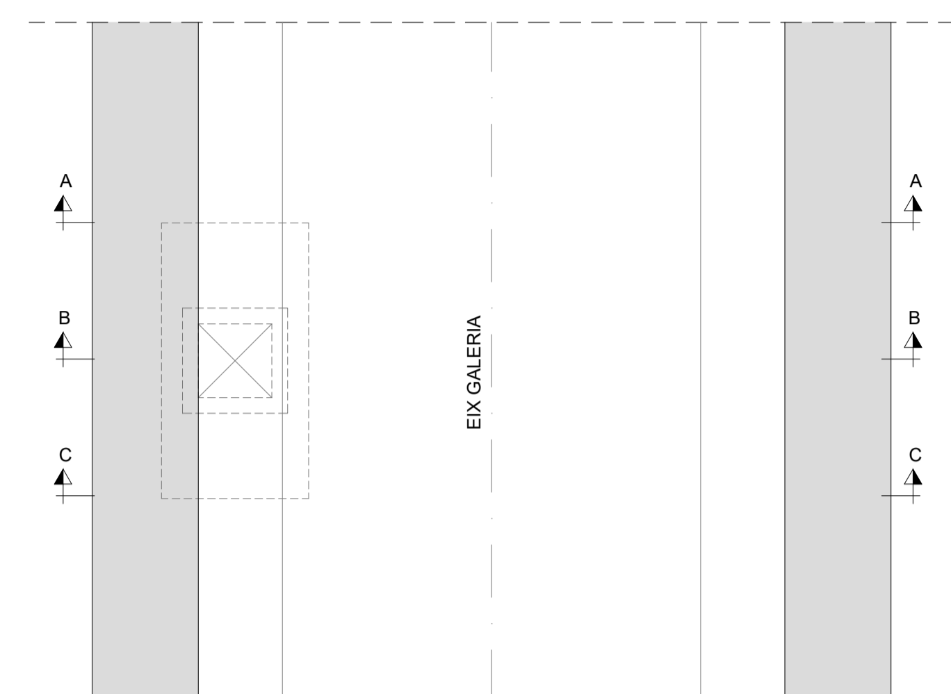
PLANTA
