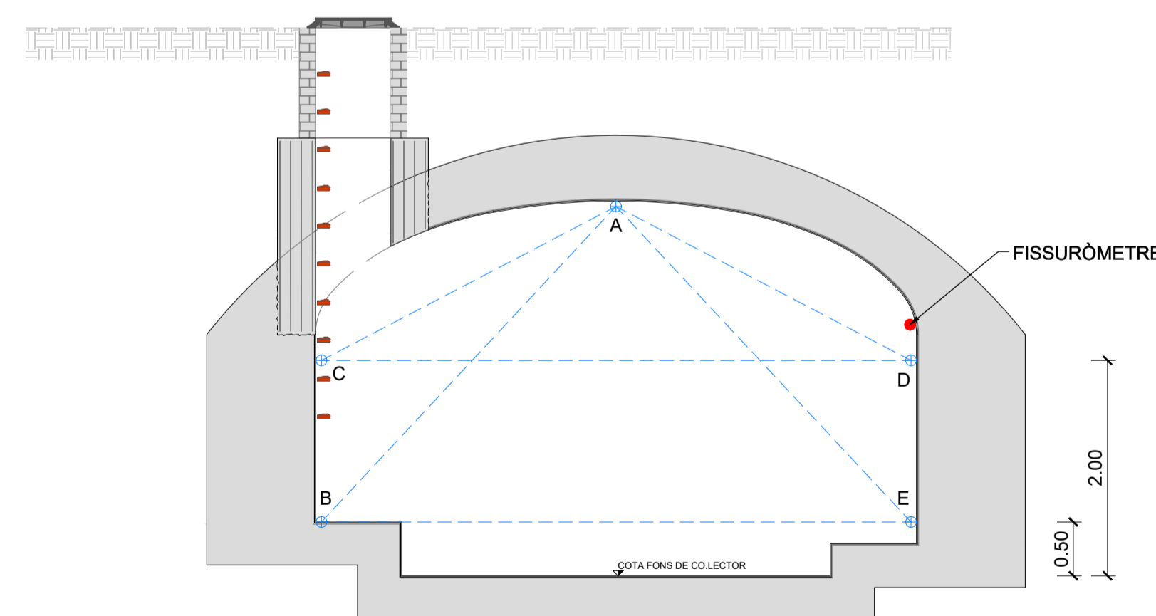
SECCIÓ B-B
