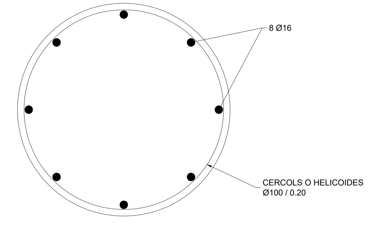
DETALL 1: ARMAT PILONS ESCALA A3 1:100
