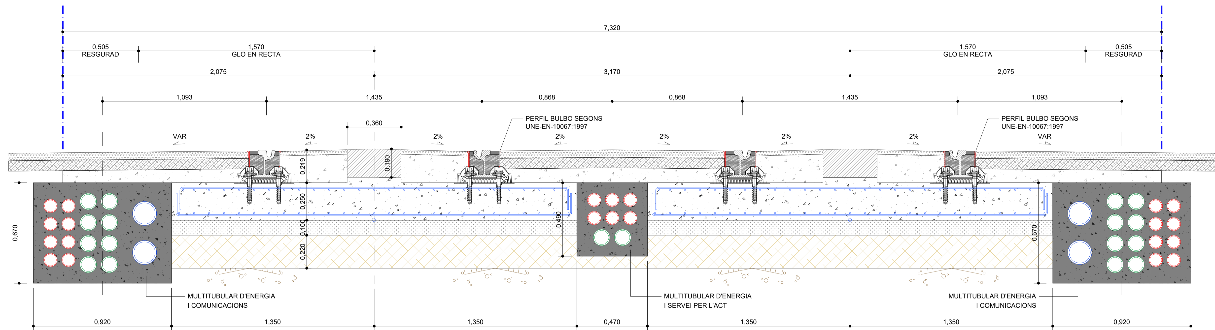
SECCIÓ NORMAL SECCIÓ ACABATS EN CREUAMENTS VIA DOBLE ESC. 1:12.5
