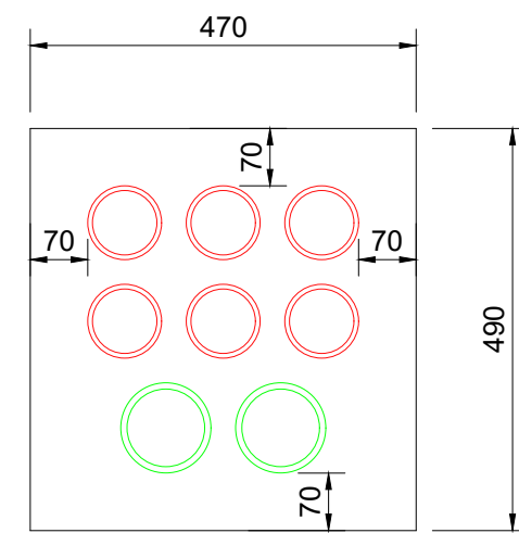
STT-01A ESC. 1/10
