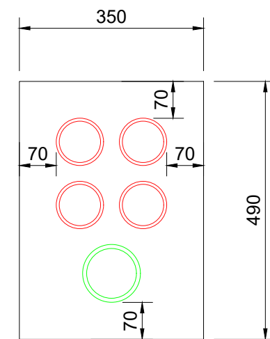
STT-02A ESC. 1/10
