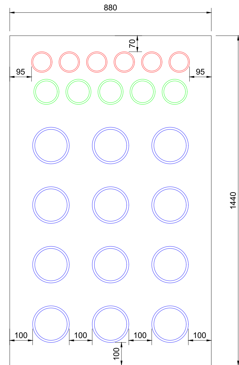
STM-07A ESC. 1/10
