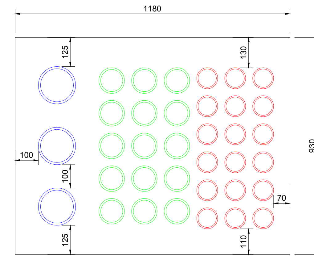
STM-10B ESC. 1/10
