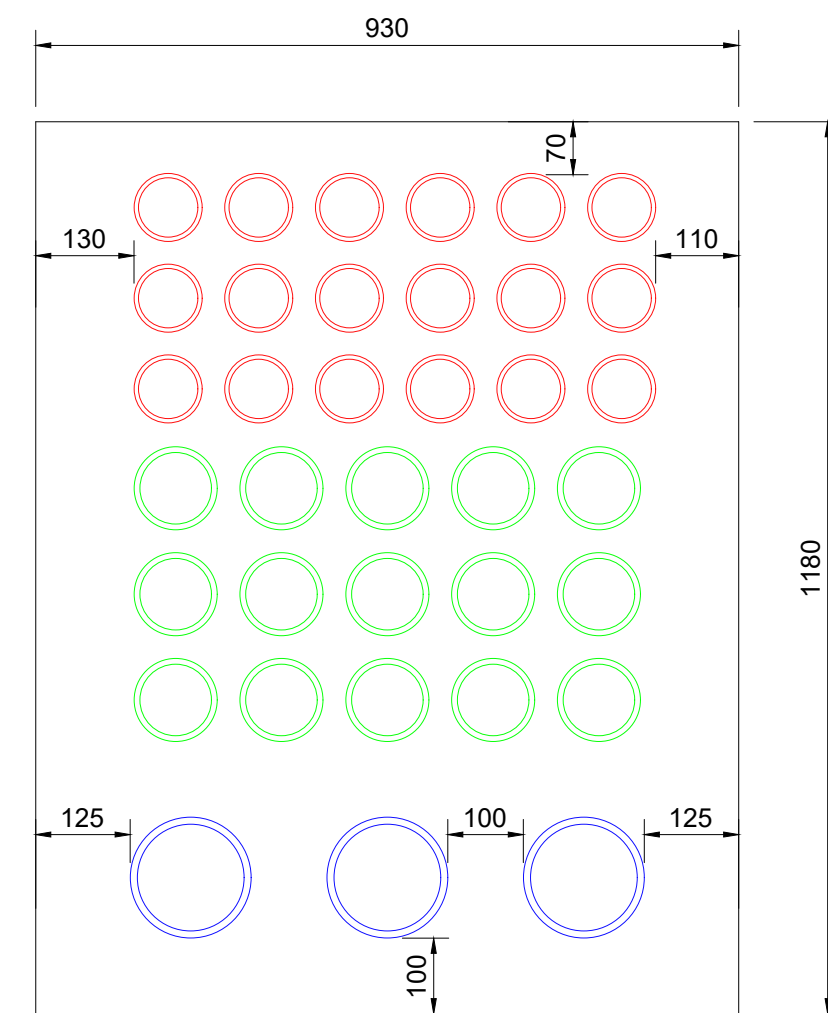
STM-10A ESC. 1/10
