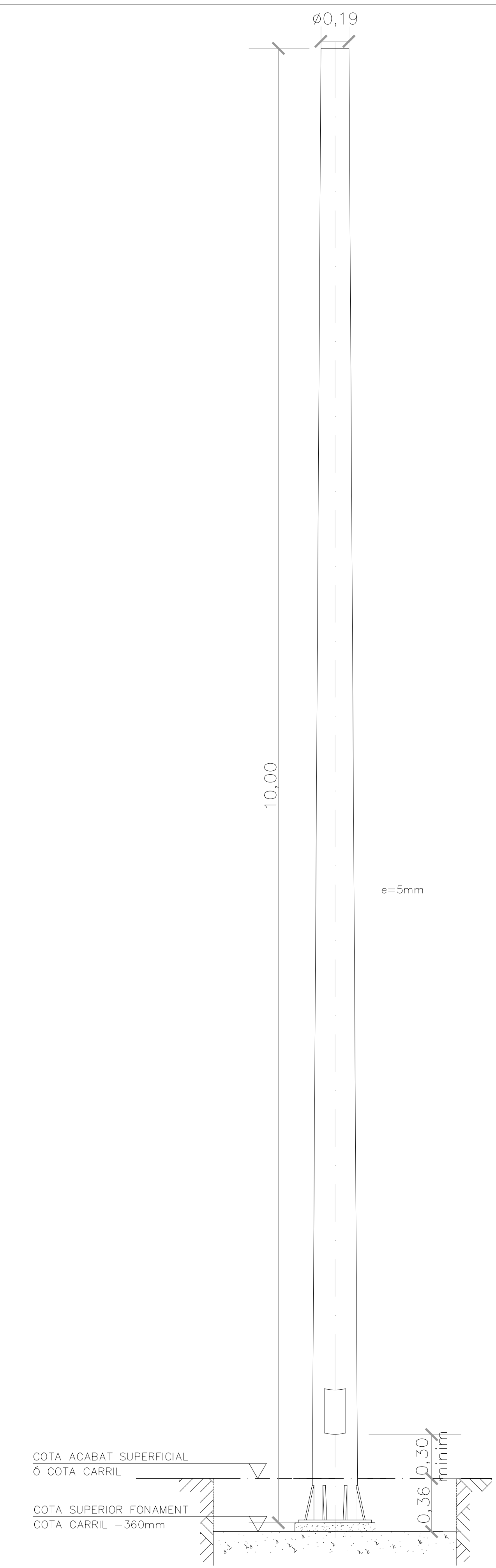
PAL TRONCOCONIC TIPUS 1-10 (Ø310 h=10.00m). PAL TRONCOCONIC TIPUS 1-9 (Ø310 h=9.00m).
