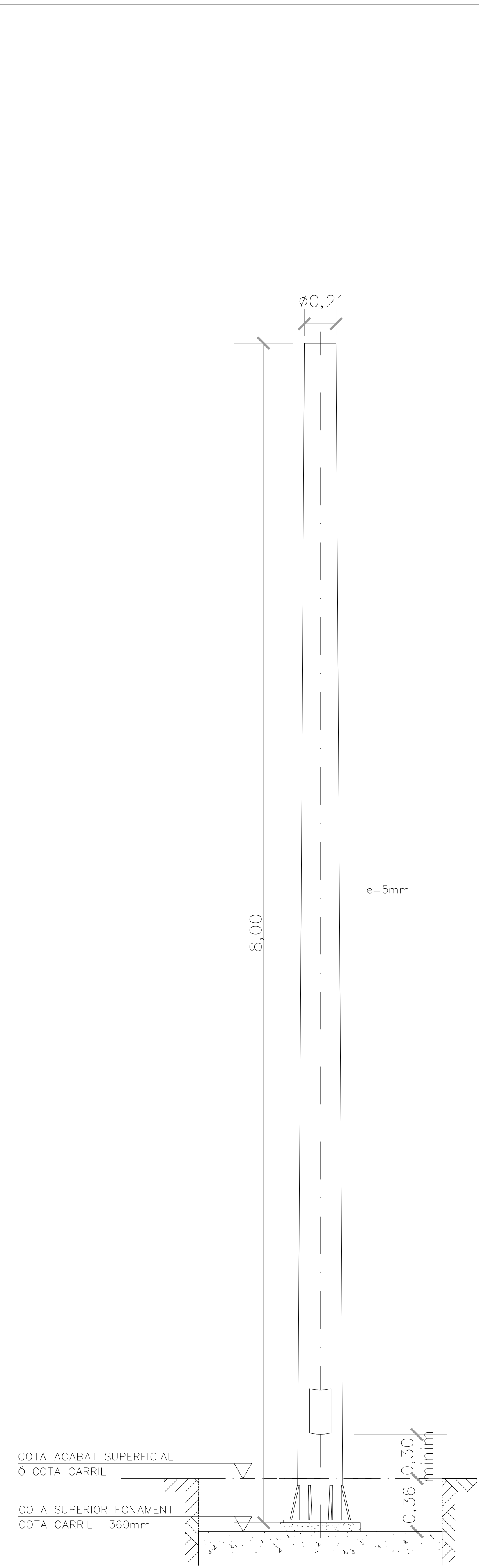
PAL TRONCOCONIC TIPUS 1 (Ø310 h=8.00m).
