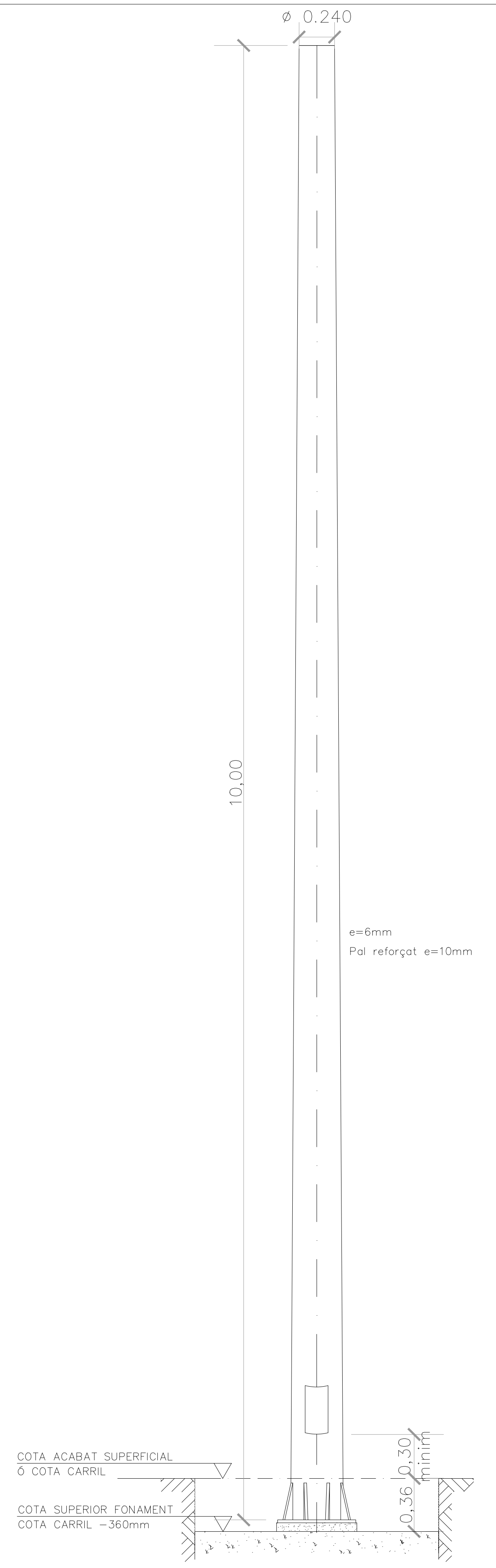
PAL TRONCOCONIC TIPUS 2-10 (Ø360 h=10.00m). PAL TRONCOCONIC TIPUS 2-9 (Ø360 h=9.00m).
