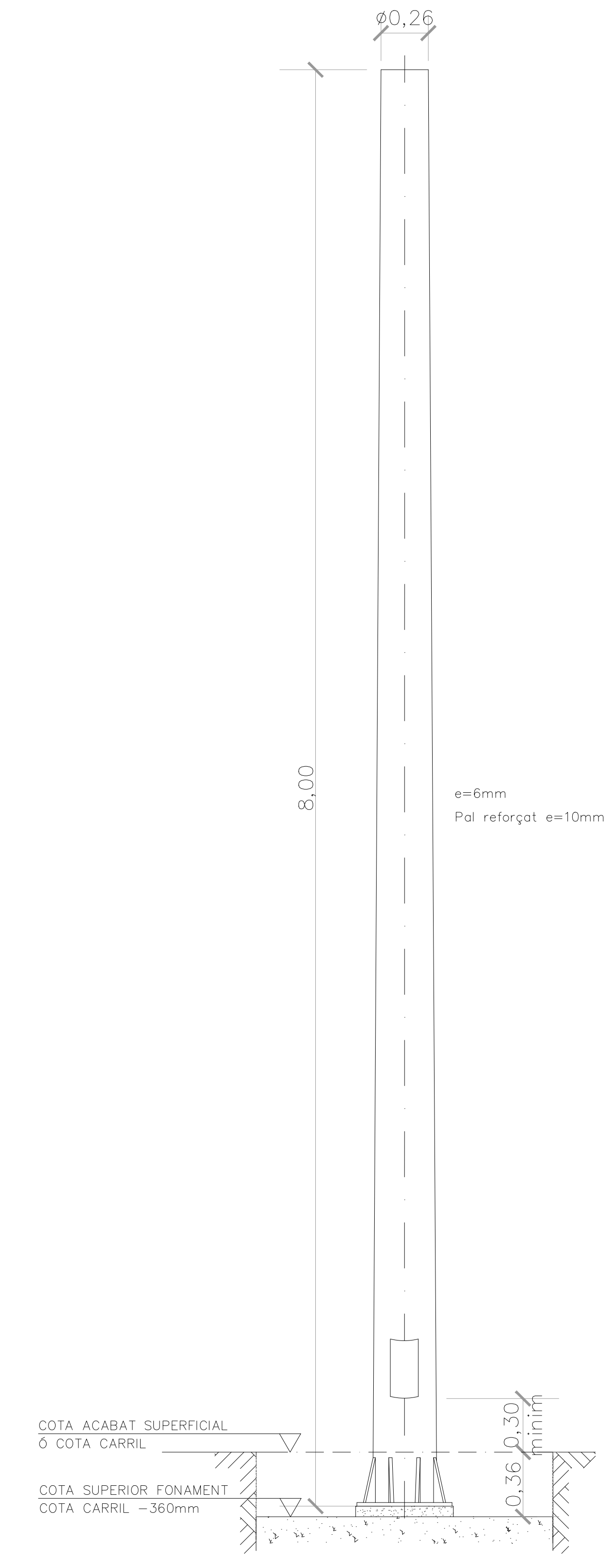
PAL TRONCOCONIC TIPUS 2 (Ø360 h=8.00m).
