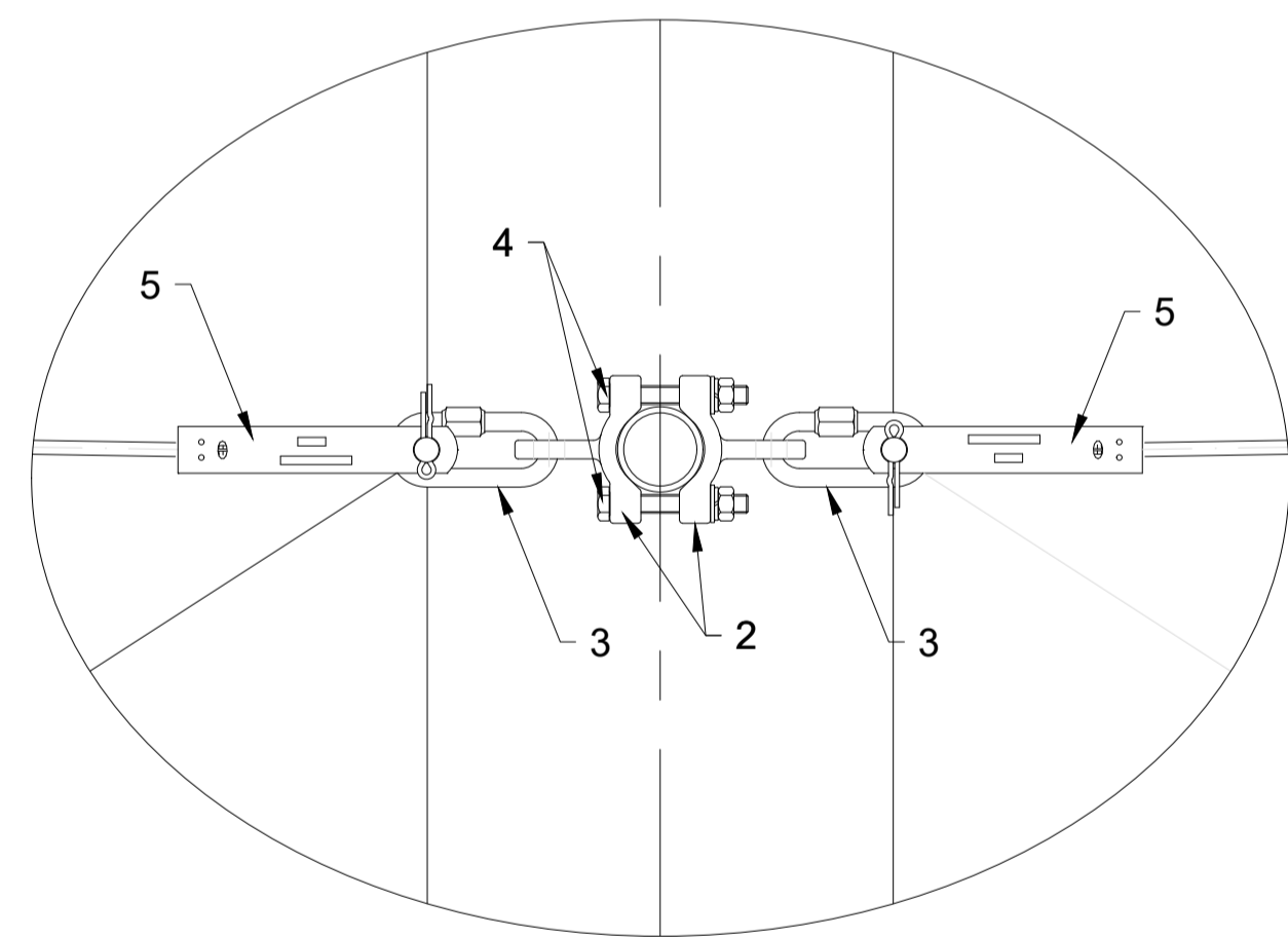
DETALL B
