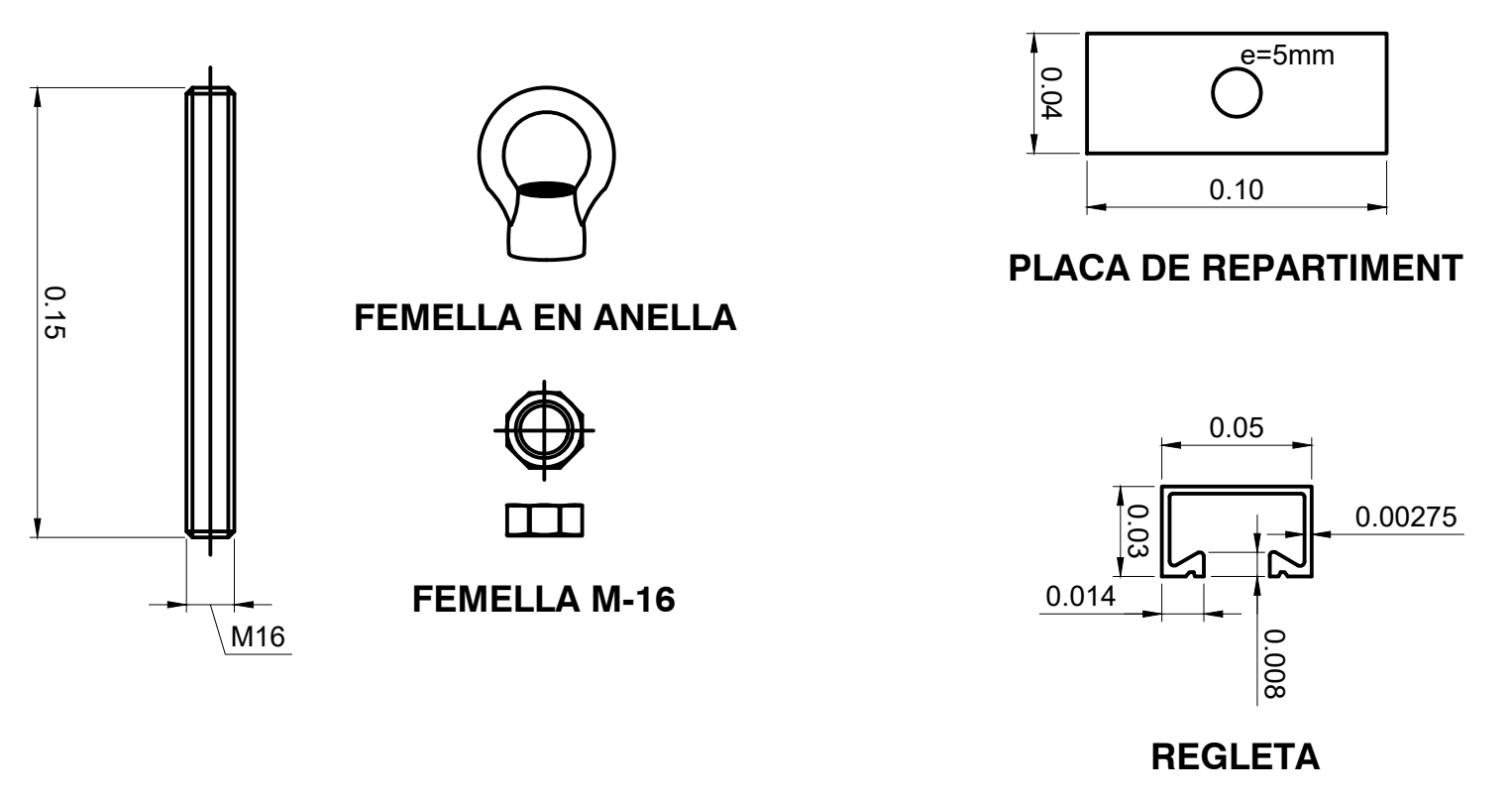
SUPORT ENGANXAMENT DE CORRIOLA Escala 1:2.5
